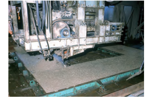
コンクリートパネルを工場生産。
